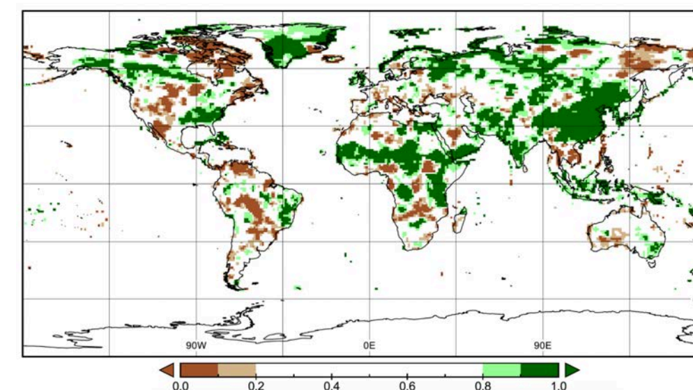
Précipitations totales sur la période de janvier à septembre 2020 exprimées comme un centile des données issues de la chronologie de référence 1951-2010.
